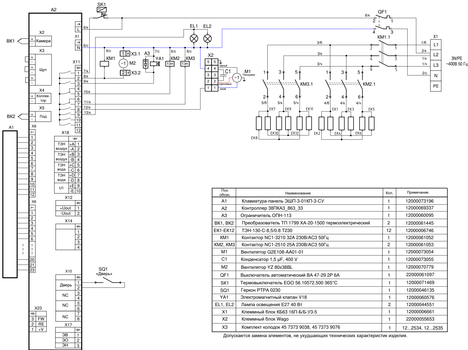
Рис.7 Схема электрическая принципиальная ЭСП-1-01КП 3EN Super
